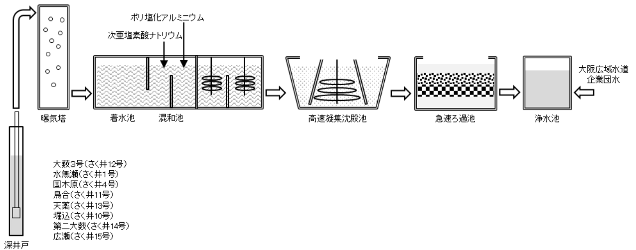
図1 大藪浄水場の処理フロー
