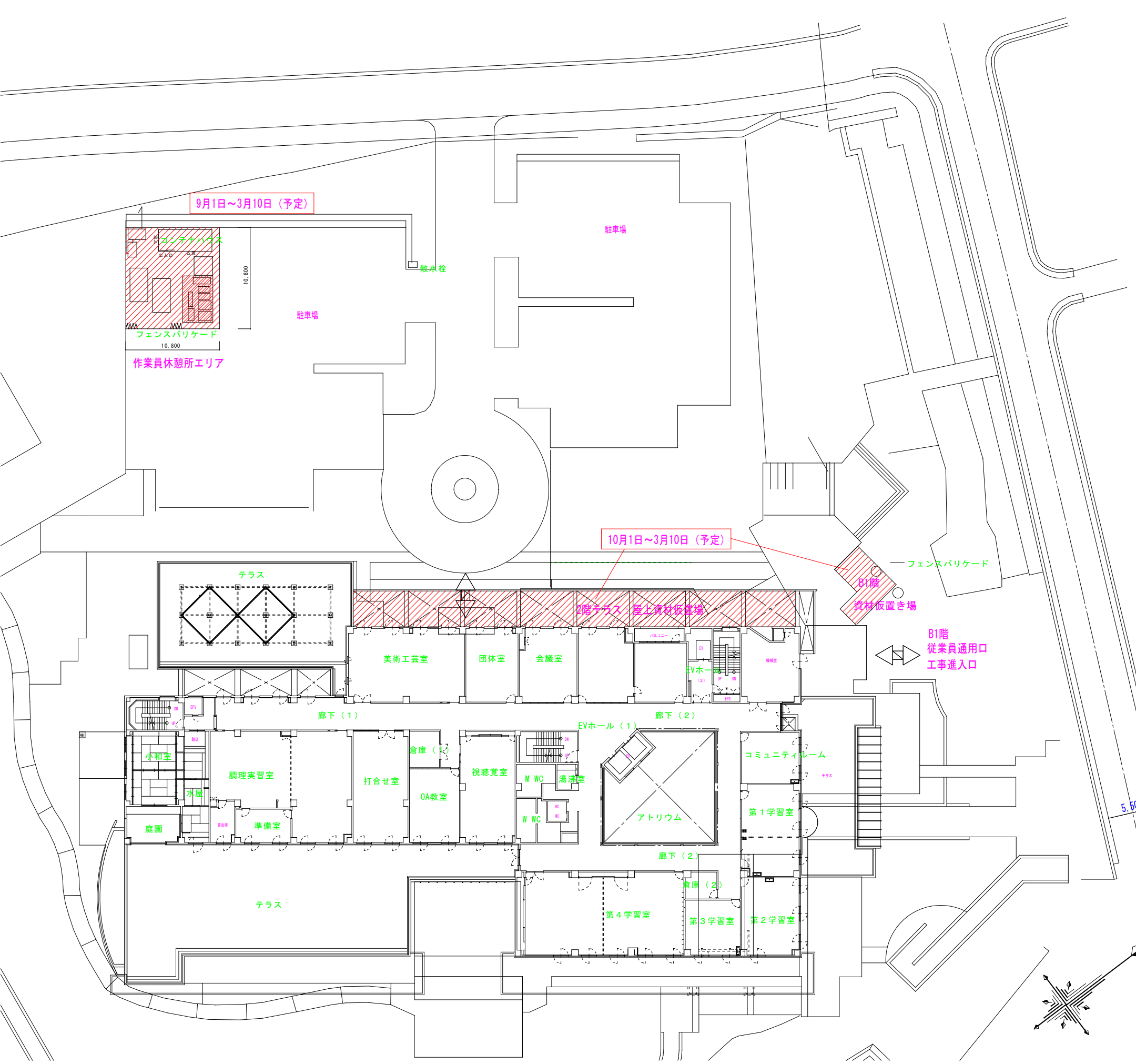
総合仮設計画図
