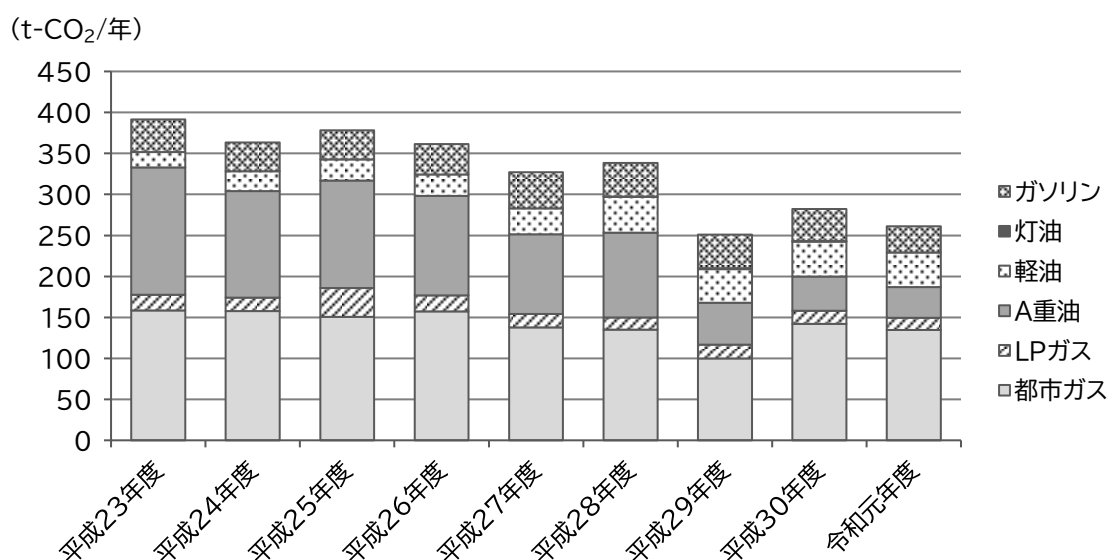
図 5-2 燃料別 CO 2 排出量
