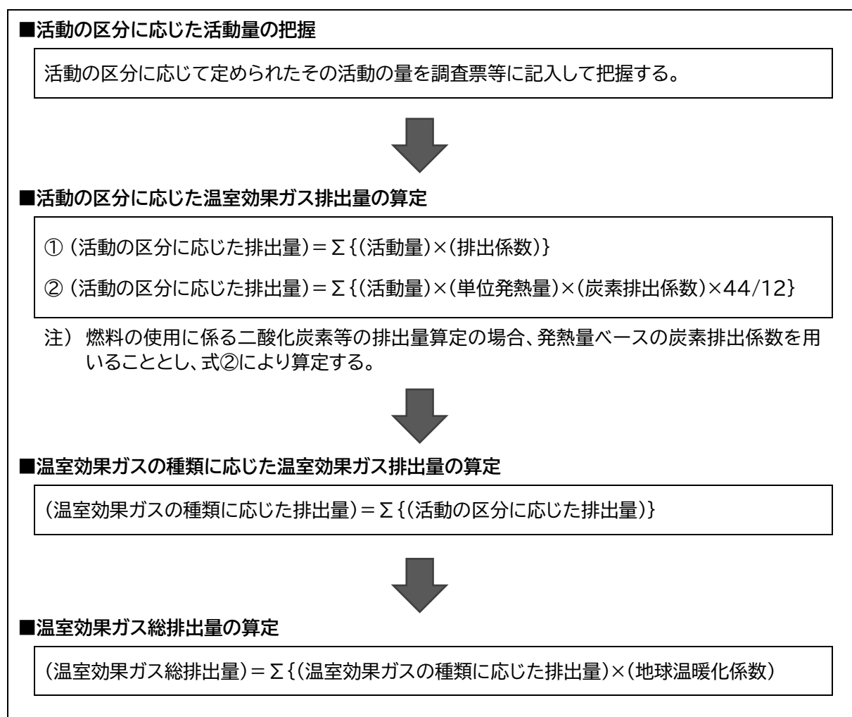
図2-2 温室効果ガス排出量の算定方法
